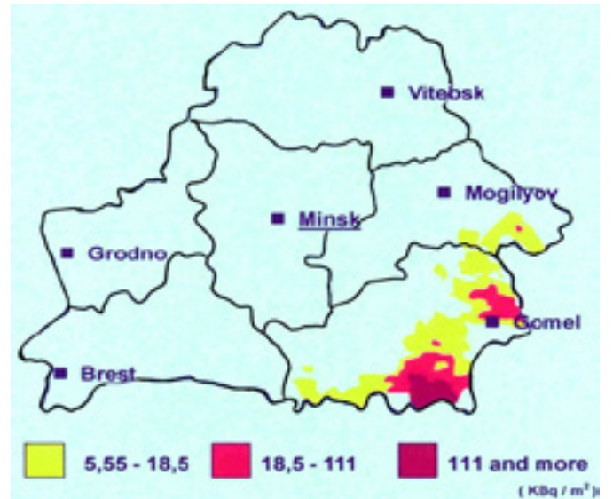
Abbildung 3-4: Verteilung SR – 90
