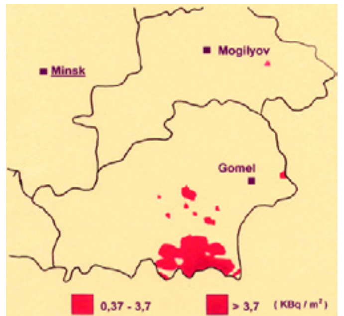
Abbildung 3-5: Verteilung PU 238, 239, 240
