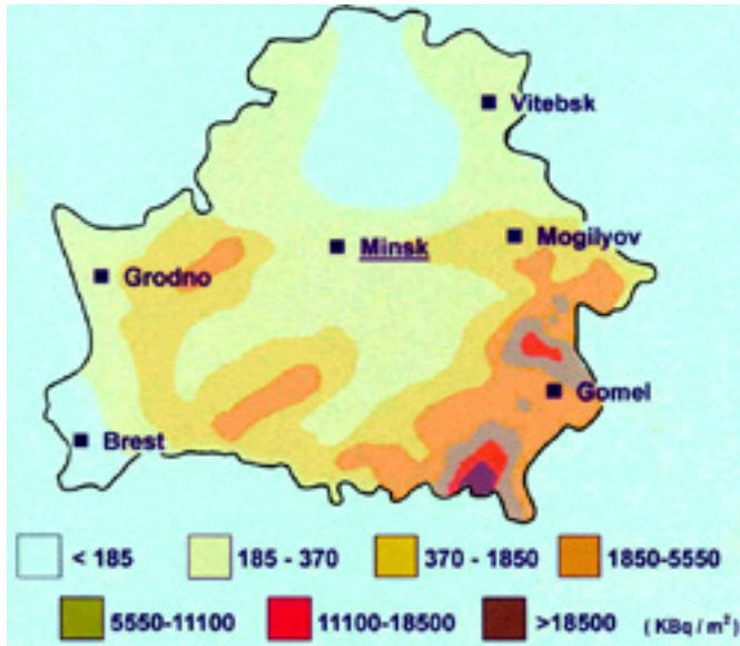
Abbildung 3-2: Jod 131 Kontamination
