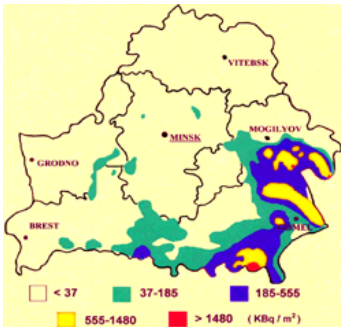
Abbildung 3-3: Verteilung Caesium
