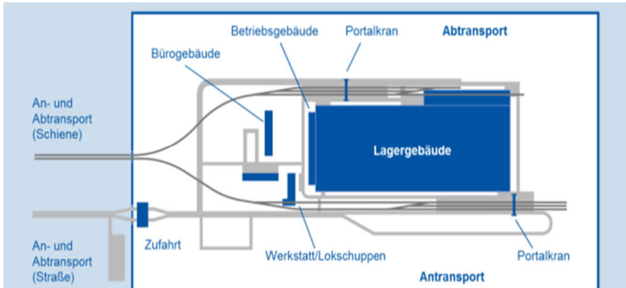
Abbildung H-3: Schematische, standortunabhängige Darstellung des Lageplans des LoK (Bildrechte: BGZ)
